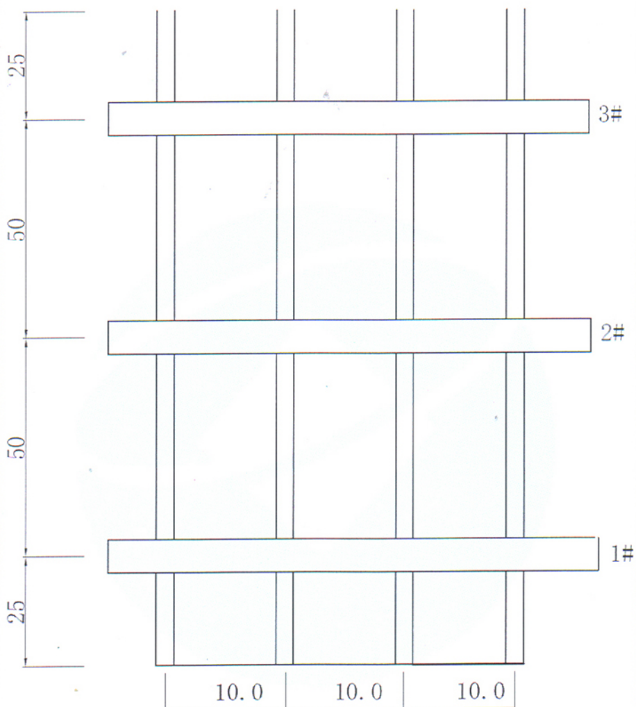
短路耐受强度试验试品安装示意图
